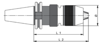
DIN-69880 VDI 3425/2
