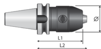
DIN-2080
