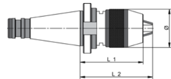
CAT-ANSI
