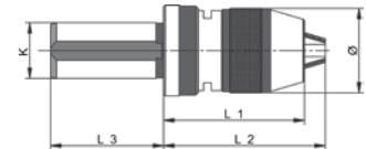
DIN-69893-A [HSK]
