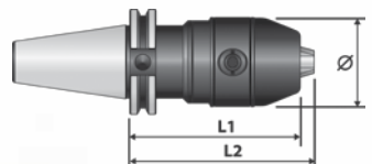
CAT-ANSI
