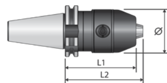
MAS-BT
