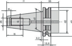
DIN 69871 (SK) ISO 30/40/50
