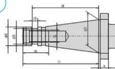
DIN 2080 ISO 30/40/50
